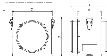
Свободное пространство для замены фильтра
