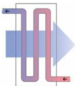
Направление потоков воды и воздуха должны быть взаимно противоположными.
