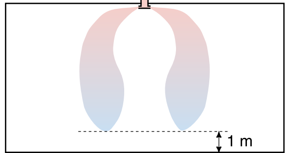
Рис. 22. Вертикальная подача воздуха потолочного диффузора
