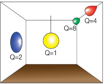
Рис. 1. Коэффициенты направленности для различно расположенных источников шума
