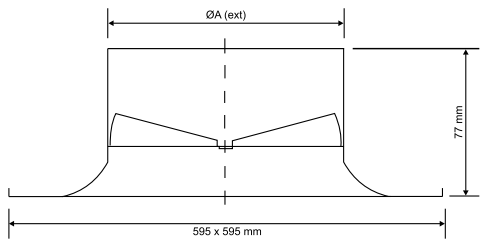
Размеры CRS-T
