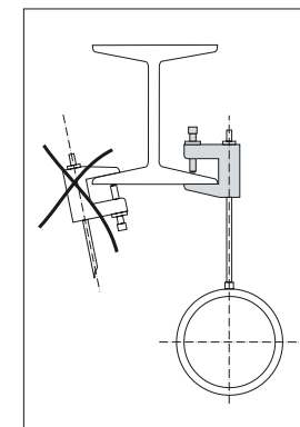
Крепление при помощи струбцины
