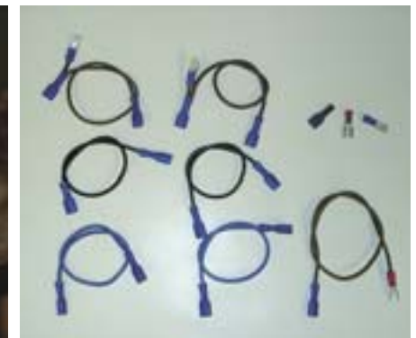
Фото 2. Провода, необходимые для подключения
